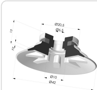
Ventosa Piatta Serie 90 Ø 42,3MM
