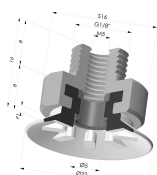
Ventosa Piatta Serie 90 Ø 22MM
