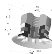
Ventosa Piatta Serie 90 Ø 22MM
