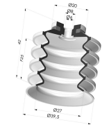
Sauggreifer 4.5 Falten Serie 92 Ø 40MM
