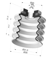
Sauggreifer 4.5 Falten Serie 92 Ø 30MM
