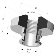
Abtrennbarer Halter IG 1/8G Produktreferenz: 9G18-2
