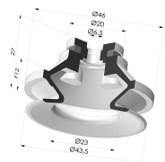
Sauggreifer 1.5 Falten Serie 91 Ø 40MM Produktreferenz: 91 40-- A
