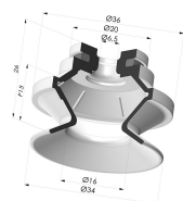
Sauggreifer 1.5 Falten Serie 91 Ø 34MM
