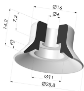
Flachsauggreifer Serie PFG Ø 25.8 mm
