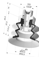
Sauggreifer 2.5 Falten Serie 96 Ø 52MM
