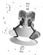
Sauggreifer 1.5 Falten Serie 91 Ø 31.8MM
