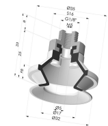
Sauggreifer 1.5 Falten Serie 91 Ø 31,8MM
