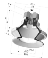
Sauggreifer 1.5 Falten Serie 91 Ø 31.8MM
