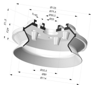
Sauggreifer 1.5 Falten Serie 91 Ø 114MM
