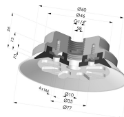
Flachsauggreifer Serie 90 Ø 75MM
