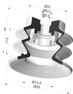
Sauggreifer 2.5 Falten Serie 96C Ø 35MM
