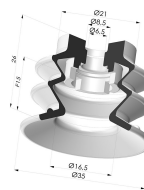
Sauggreifer 2.5 Falten Serie 96C Ø 35MM
