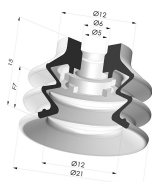
Sauggreifer 2.5 Falten Serie 96C Ø 20MM
