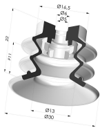
Sauggreifer 2.5 Falten Serie 96B Ø 30MM
