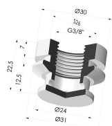
Abtrennbarer Halter IG G3/8"
