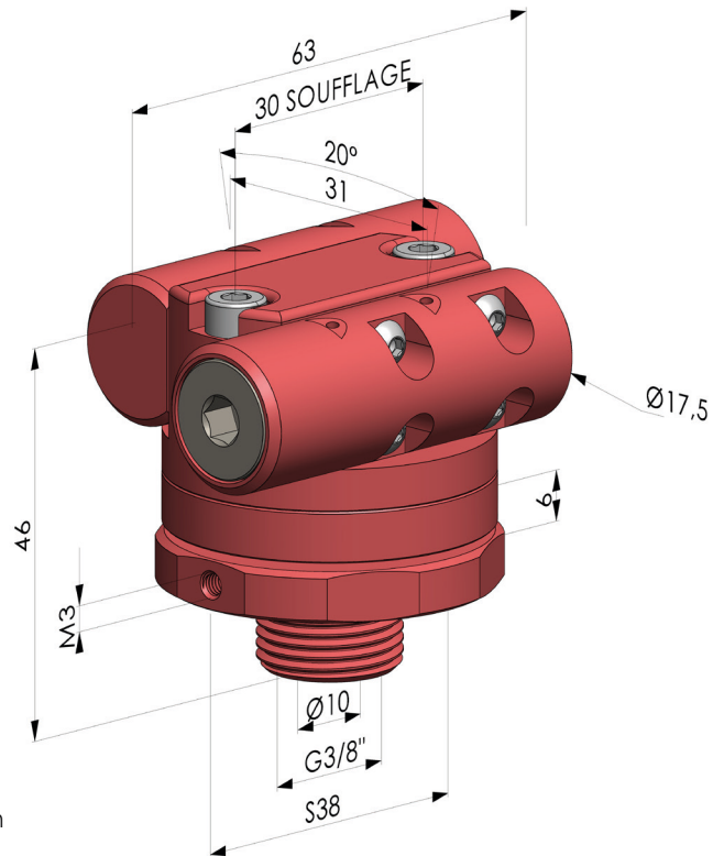
BSR 38 30 ■ Eloxiertes Aluminium Die Werte sind in MM angegeben
