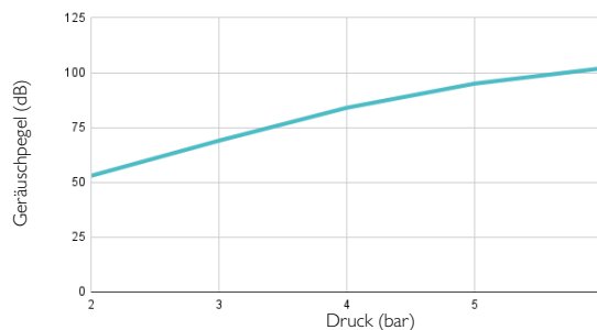
GERÄUSCHPEGEL
