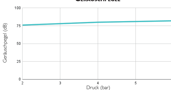
GERÄUSCHPEGEL
